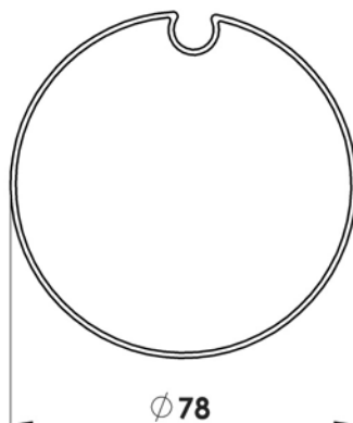
Cilindro d'avvolgimento (6-011084)
