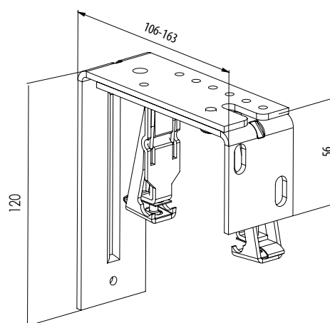
Supporto regolabile (gancio interno Fe Click) 106-163 mm P 009/1 (2-00404) (per il profilo superiore 56 x 58)
