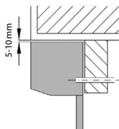
Montaggio nella facciata
