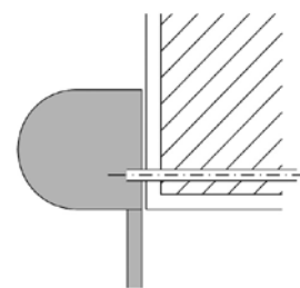
Montaggio sulla facciata
