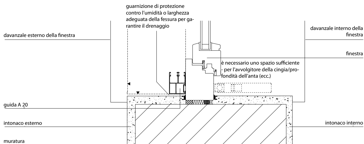
dettaglio collegamento - vista laterale (parte inferiore)
