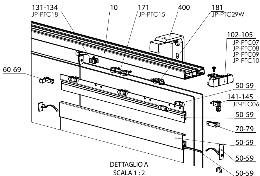
Dettaglio A
