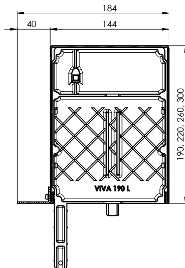
Sezione cassonetto a muro VIVA
