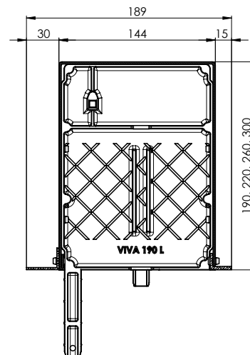
Sezione cassonetto sotto intonaco VIVA + P 020/03, P 080/03, P 081/03 190x150Lb 220x150Lb 260x150Lb 300x150Lb
