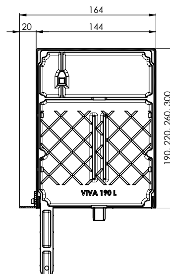
Sezione cassonetto a muro VIVA
