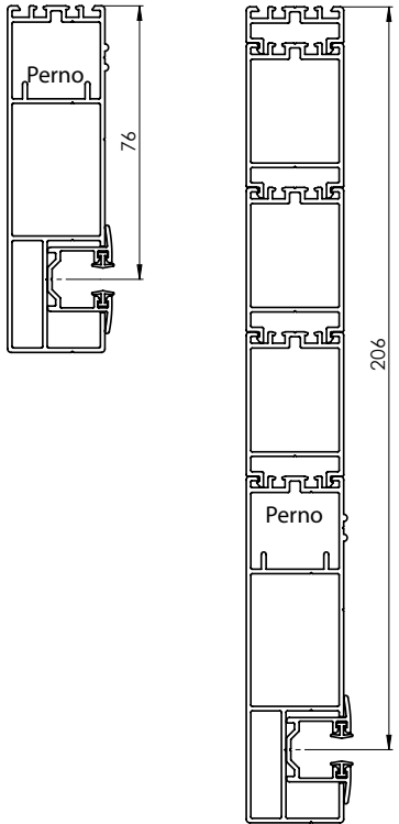
Profilo base P 081 Massima estensione possibile del profilo di base P 081
