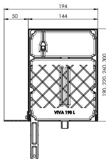
Sezione cassonetto a muro VIVA
