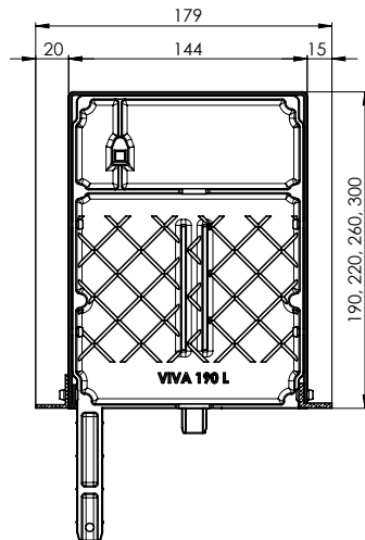
Sezione cassonetto sotto intonaco VIVA + P 020/02, P 080/02, P 081/02 190x150Lb 220x150Lb 260x150Lb 300x150Lb
