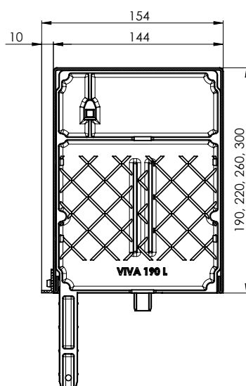
Sezione cassonetto a muro VIVA
