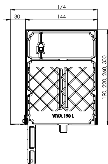
Sezione cassonetto a muro VIVA
